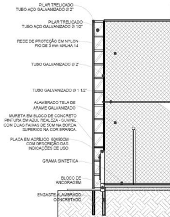
Figura 08 – Detalhe Ilustrativo de Instalação do Alambrado e Tela (Fonte: Autoria/2021)
