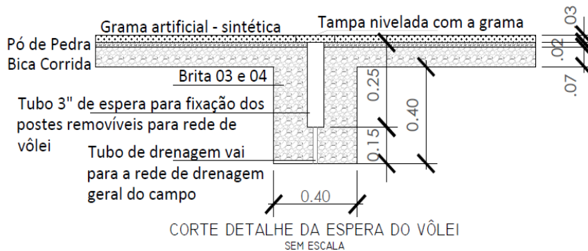
Figura 06 – Detalhe da drenagem (Fonte: Autora/2021)
