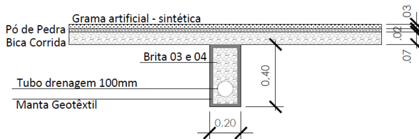
CORTE DETALHE VALA DRENAGEM SEM ESCALA
