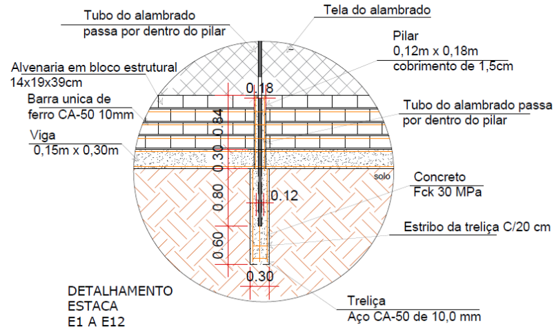
Figura 05 – Detalhamento de estaca (Fonte: Autora/2021)
