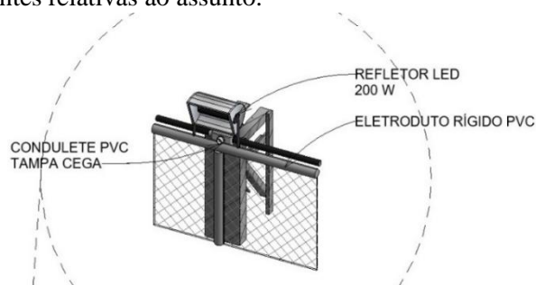
Figura 10 – Detalhe Ilustrativo de Instalação Refletor (Fonte: Autora/2021)
